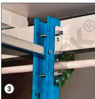
Doppelgeschossanlage zur Lagerung von Reifen.
